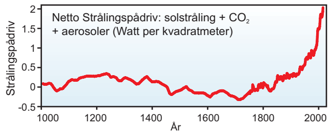
Kombinert strålingspådriv fra variasjoner i solstråling, CO 2 og aerosoler – de kortvarige effektene til vulkaner er utelatt. 38
