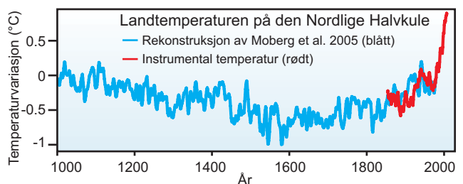
Temperaturrekonstruksjon på den nordlige halvkule (blått) pluss instrumentale målinger av landtemperaturen på den nordlige halvkule (rødt). 21
